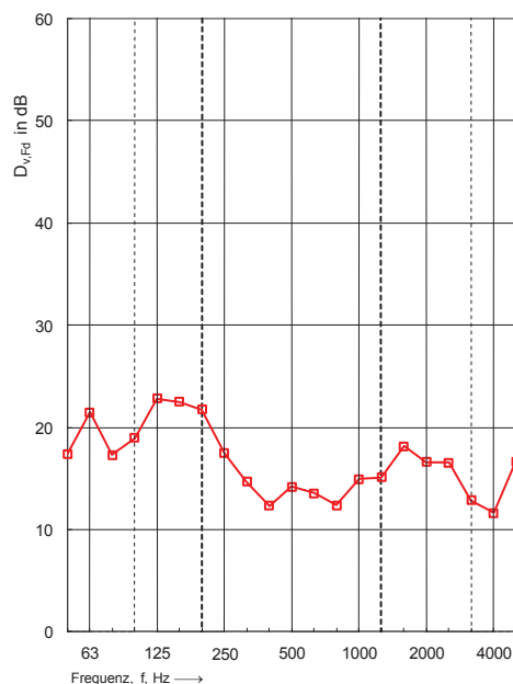
Abbildung 21 D_{v,ij} , K_{ij} : Horizontaler T-Stoß – Hohlkastendecke durchlaufend, Flanke beschwert: Messdaten D_{v,Fd} mit zugehörigen Messkurven (links), Messdaten K_{Fd} mit zugehörigen Messkurven (rechts)
