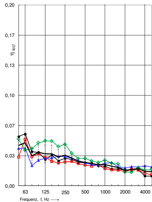
Abbildung 2 \eta_{\text{tot}} : Horizontaler T-Stoß – BSP Decke durchlaufend, Trennbauteile z.T. mit Beplankung, Messdaten \eta_{\text{tot},F} mit zugehörigen Messkurven (links), Messdaten \eta_{\text{tot},f} mit zugehörigen Messkurven (rechts)
