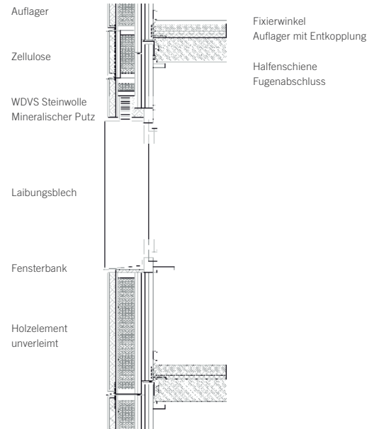
ANGEHÄNGTE 15,5 CM NUR-HOLZ WAND MIT ZUSÄTZLICHER DÄMMUNG.
